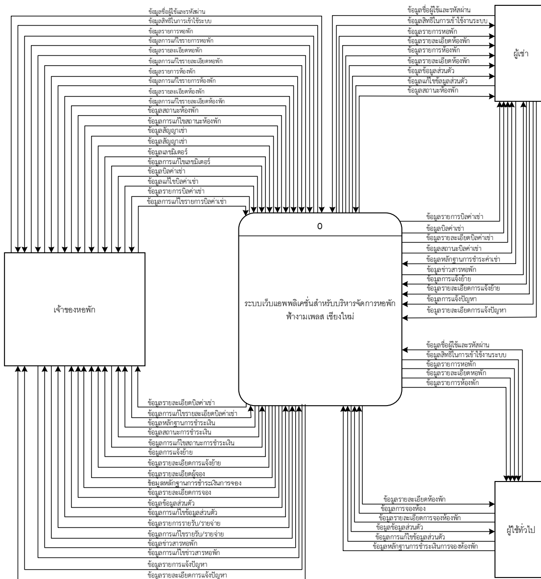
ภาพที่ 3.6 แผนภาพบริบท (Context Diagram)
