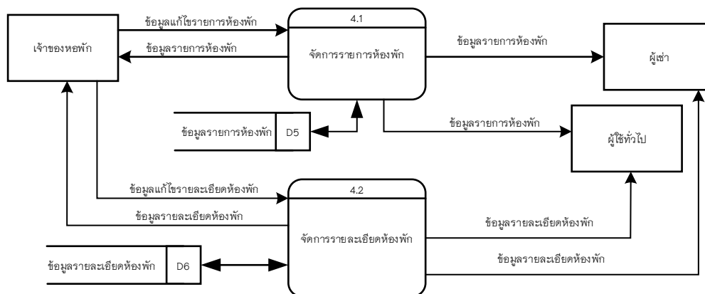
ภาพที่ 3.9 แผนภาพกระแสข้อมูลระดับที่ 4.0 จัดการห้องพัก
