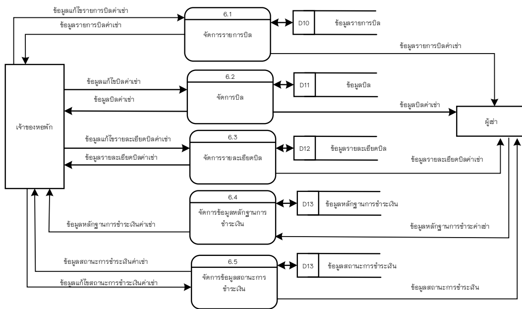
ภาพที่ 3.10 แผนภาพกระแสข้อมูลระดับที่ 6.0 การทำบิล
