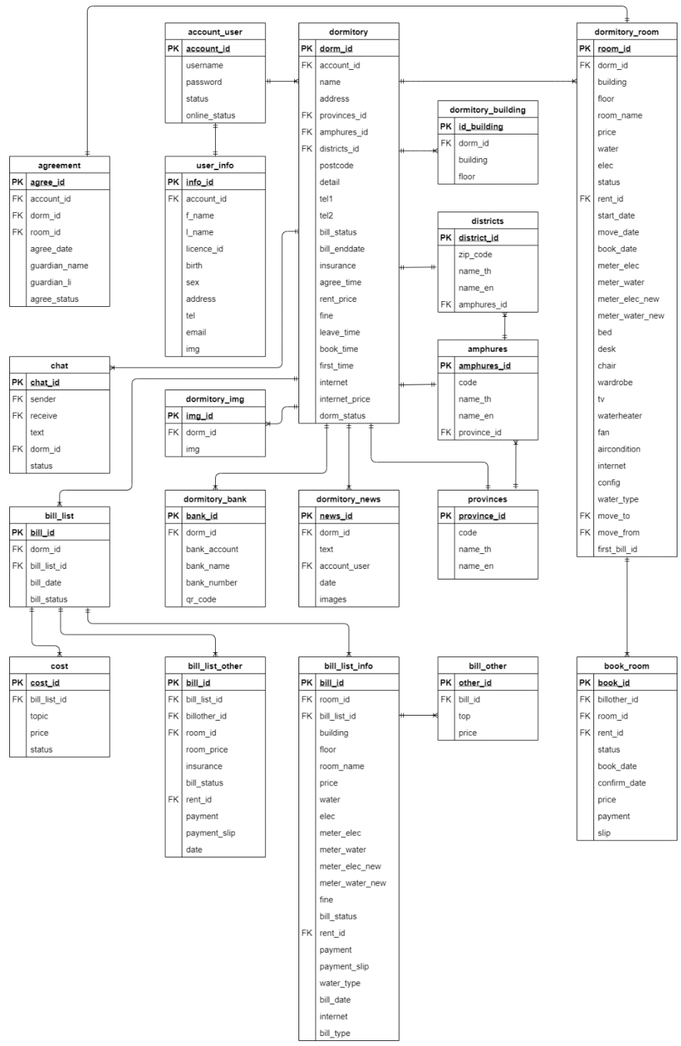
ภาพที่ 3.11 ER-Diagram
