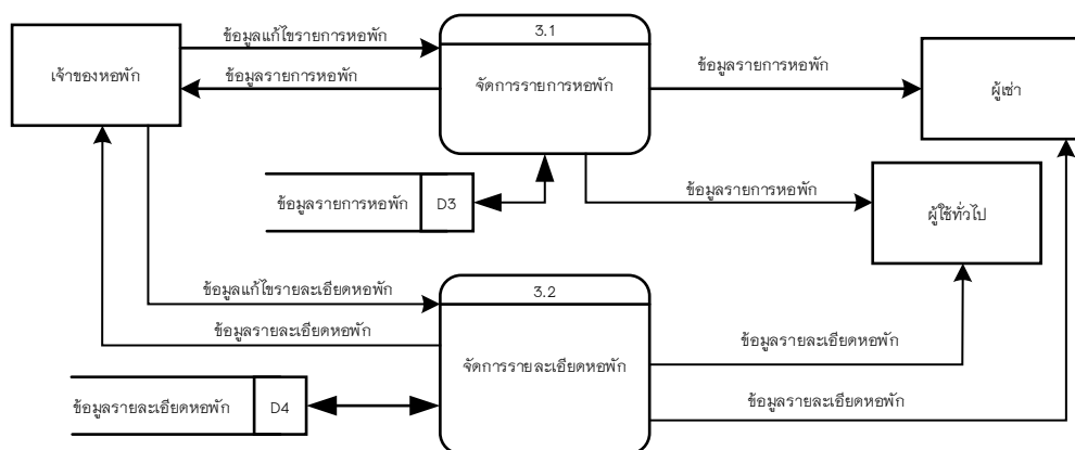
ภาพที่ 3.8 แผนภาพกระแสข้อมูลระดับที่ 3.0 จัดการห้องพัก
